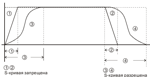
Характеристики разгона/торможения
